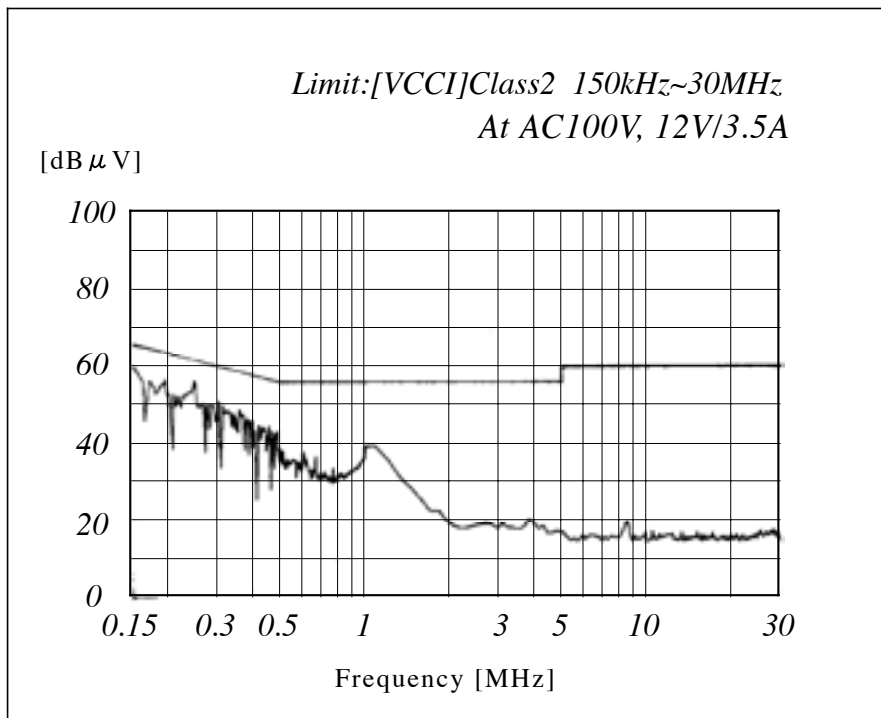
Fig.10 Input Feedback Noise
